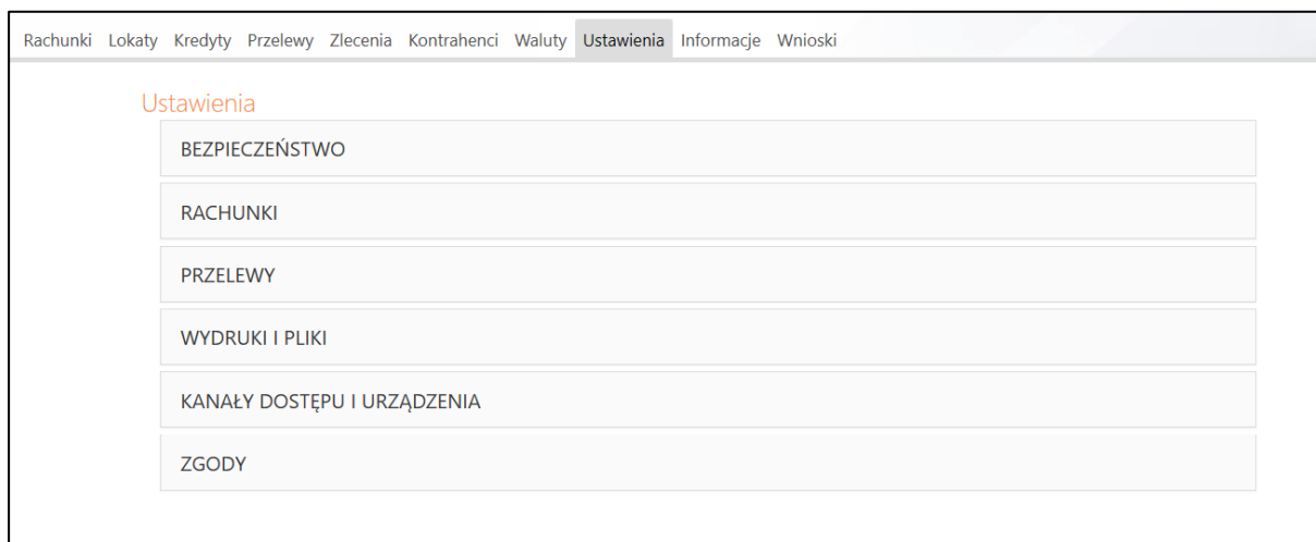
Rys. 42 Okno „Ustawienia”
